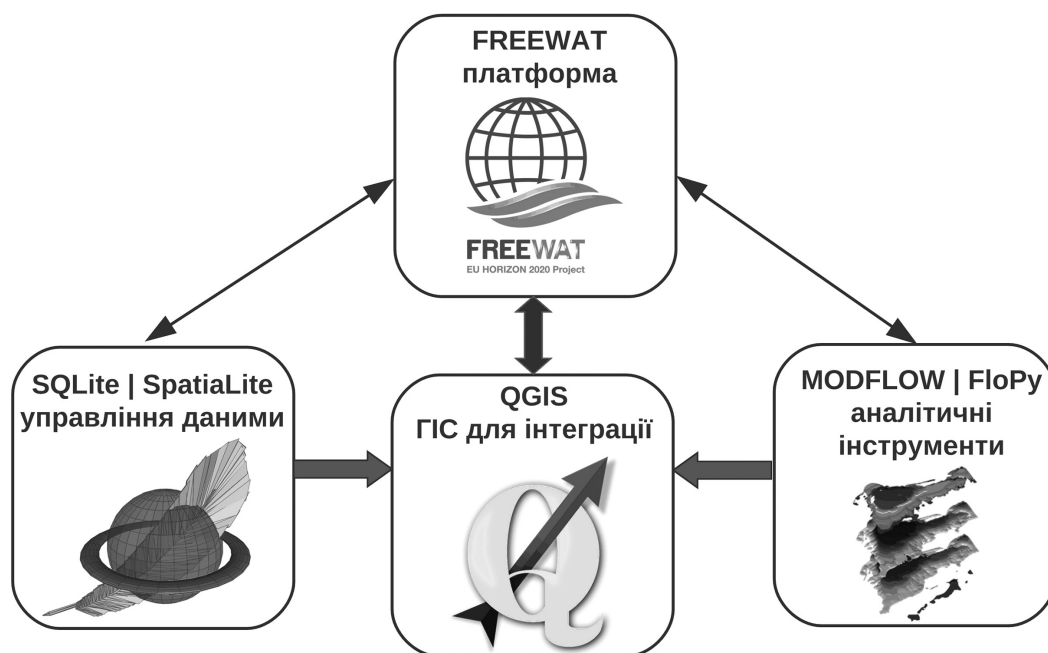
Рисунок 2. Узагальнена структура платформи FREEWAT, інтегрованої з ГІС-середовищем QGIS
